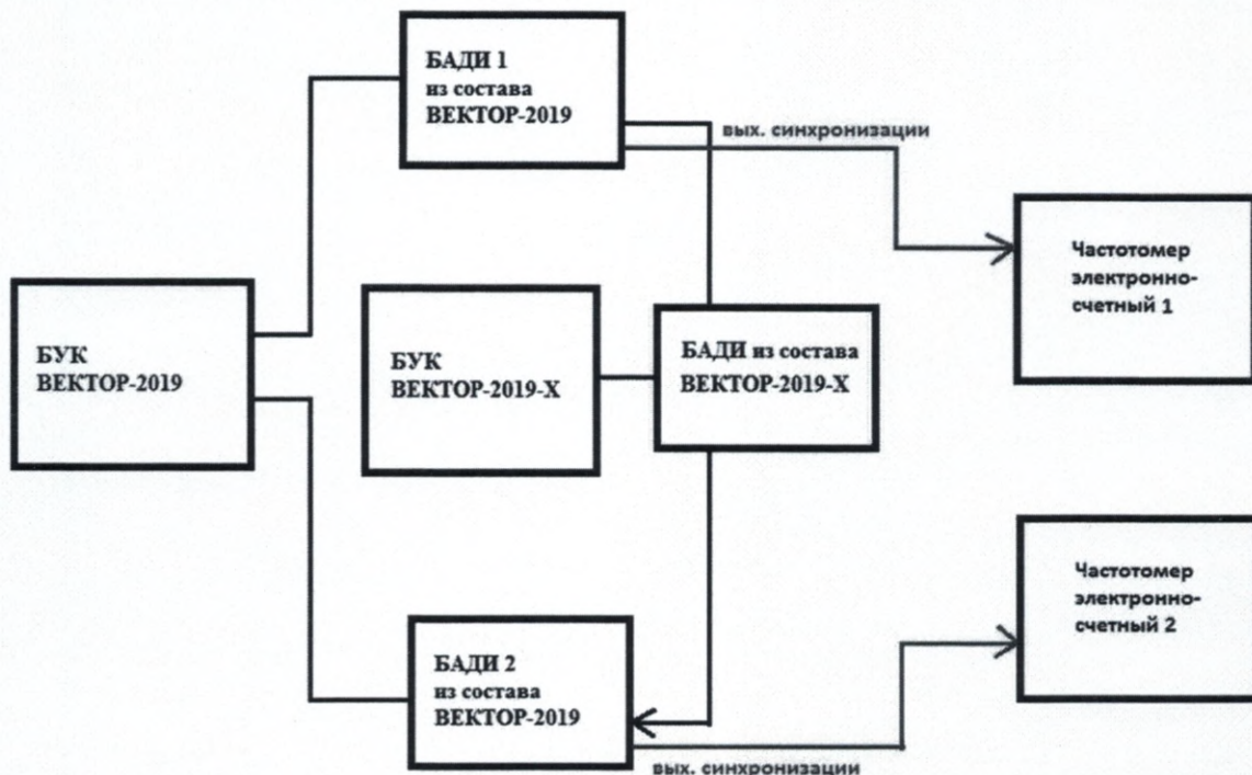
Рисунок 19 – Схема для определения диапазона и относительной погрешности измерения пропускной способности канала передачи данных
