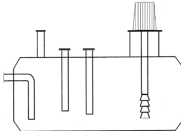
Рисунок 1 – Эскиз резервуаров РГС-25
