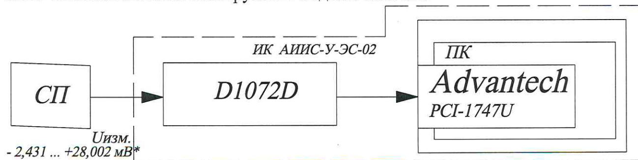
Рисунок 10.6 – Схема определения МХ ЭЧ ИК температуры газа с ПП термоэлектрического типа
