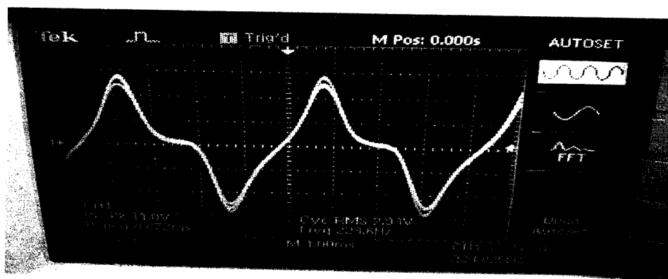
Рисунок 1 – Сигнал на выходе технически исправного ТДИ-80
