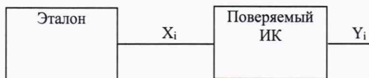
Рисунок 2 – Схема проверки ИК измерения среднеквадратического и амплитудного значения сигналов напряжения переменного тока гармонической формы
