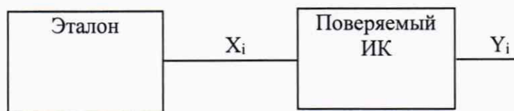
Рисунок 1 – Схема проверки ИК измерения сигналов напряжения и силы постоянного тока, сопротивления
