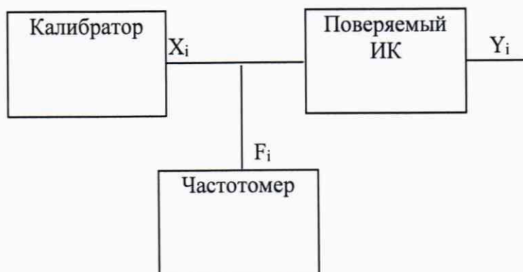
Рисунок 5 – Схема проверки ИК измерения частоты сигналов напряжения переменного тока
