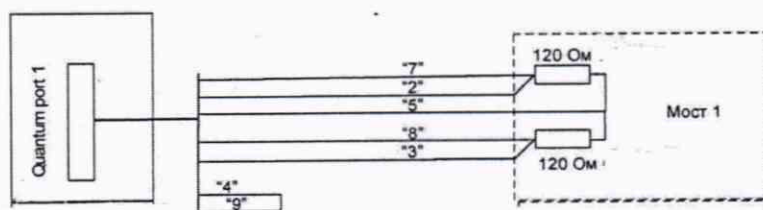
Рисунок 6 – Схема проверки ИК измерений сигналов от тензодатчиков
