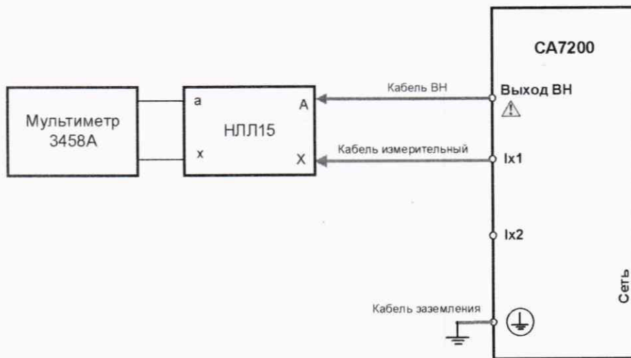
Рисунок 5 - Схема измерения испытательного напряжения свыше 1 кВ и его частоты
