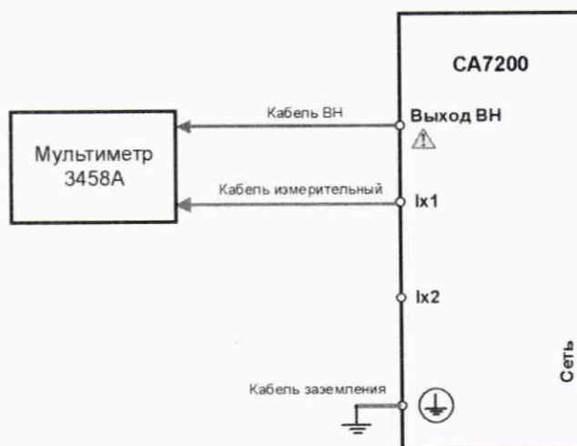
Рисунок 4 - Схема измерения испытательного напряжения до 700 В и его частоты
