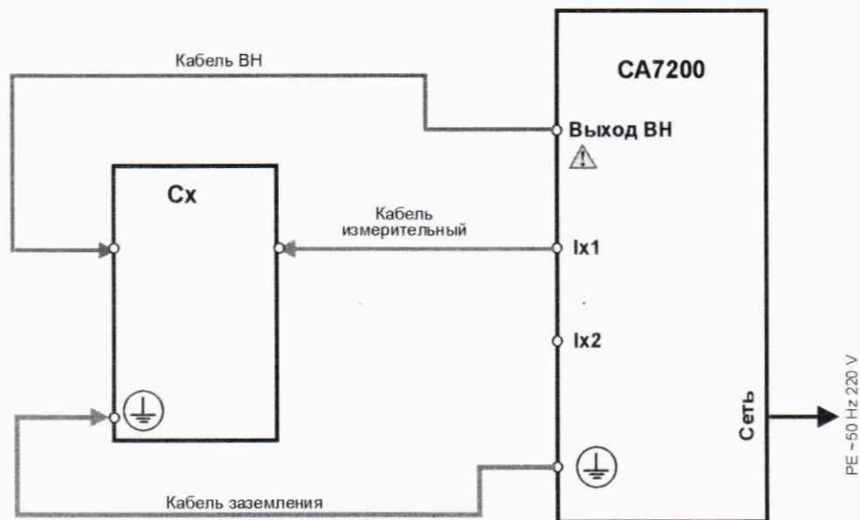
Рисунок 1 - Схема измерения электрической емкости
