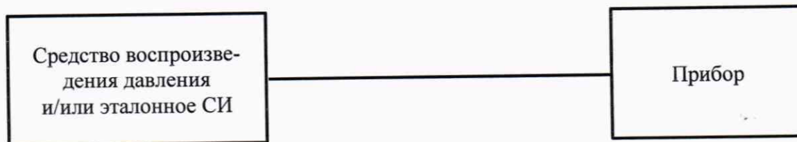
Рисунок А.1 – Схема проверки прибора при измерении давления
