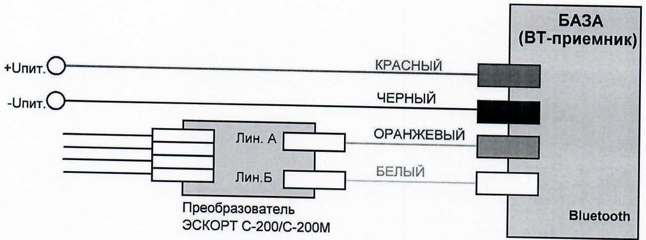
Рисунок А.1 – Схема подключения к ПК
