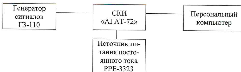
Рисунок 6.3.2 Схема подключения к АГАТ на диапазоне измерений от 200 Гц до 8000 Гц
