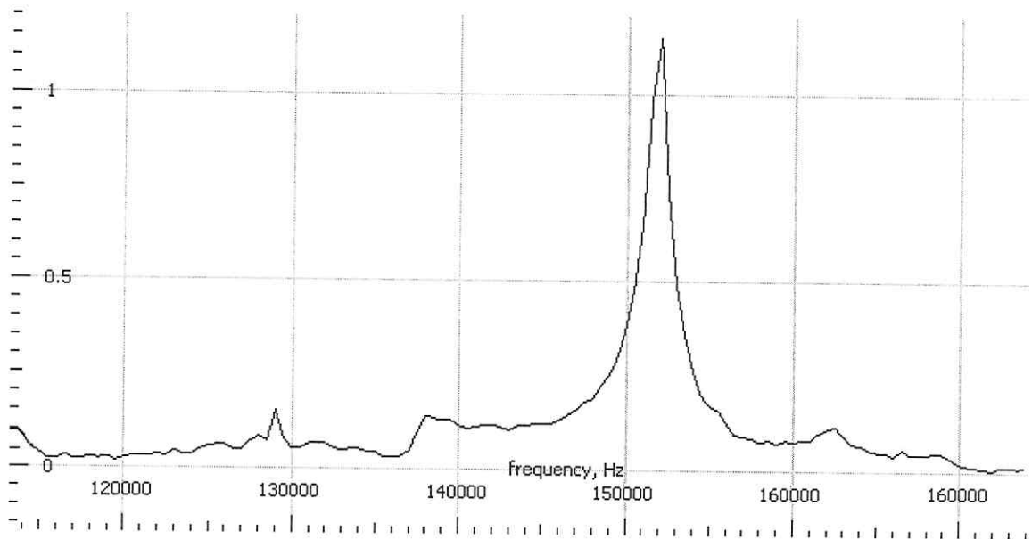
Рисунок В.3 – Спектр сигнала акселерометра 1С301НА зав. № 20058
