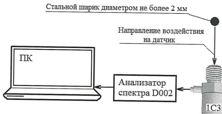
Рисунок В.1 – Схема проверки частоты установочного резонанса
