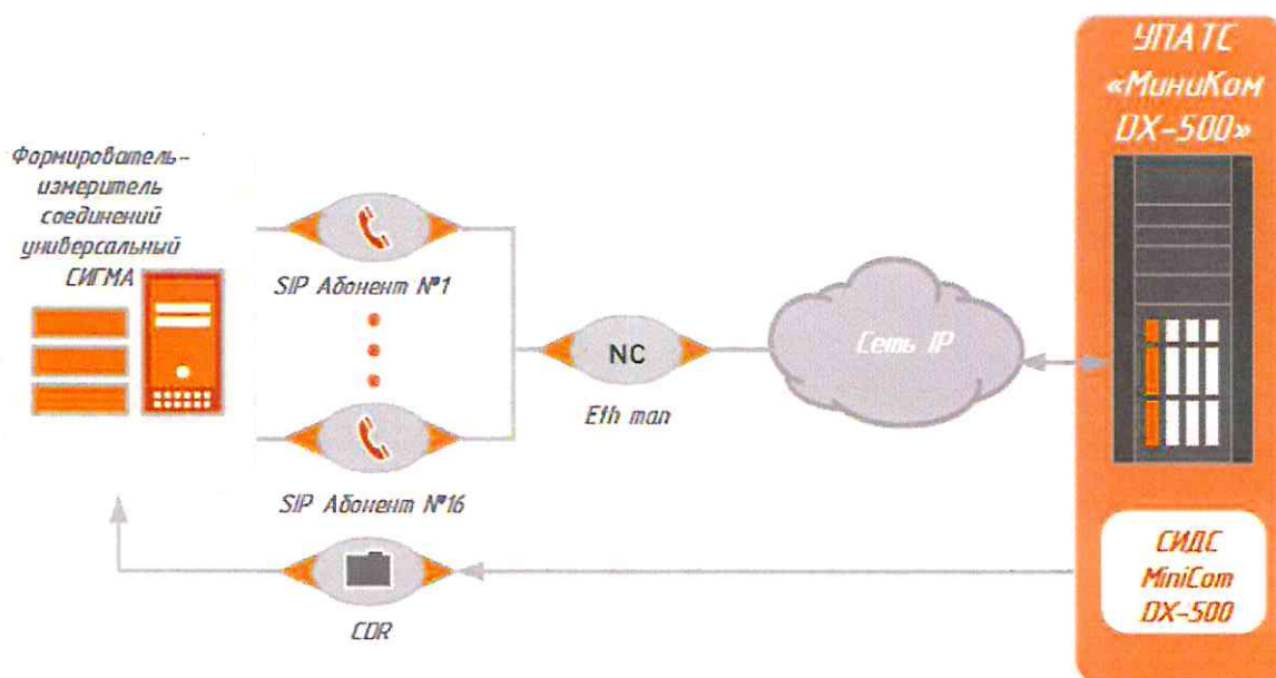
Рисунок 1- Схема поверки
