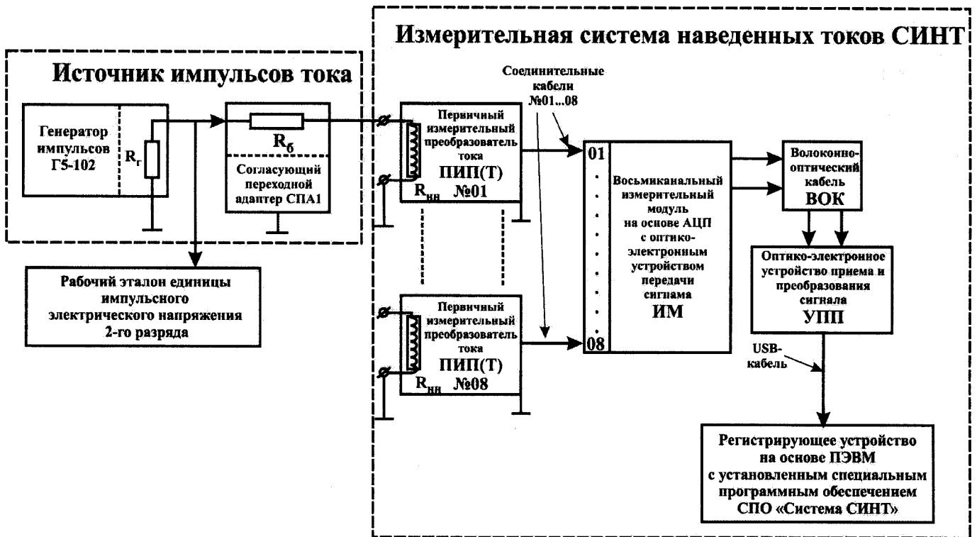
Рисунок 1 – Схема соединений при проведении измерений системы СИИТ
