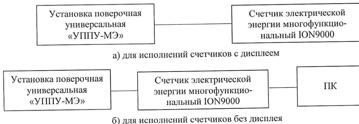
Рисунок 1 – Схемы подключений при определении метрологических характеристик счетчиков
