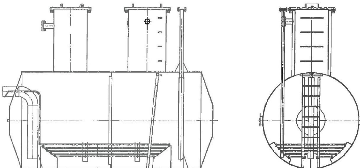
Рисунок 1 – Эскиз РГС
