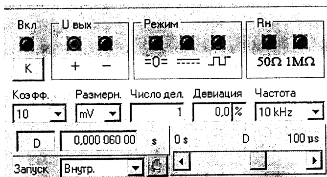
Рисунок 1 – Начальные положения органов управления на панели управления «УИ К2С-62А КУ» при измерении абсолютной погрешности измерений напряжения в режиме «ЦО ВЧ» установки
