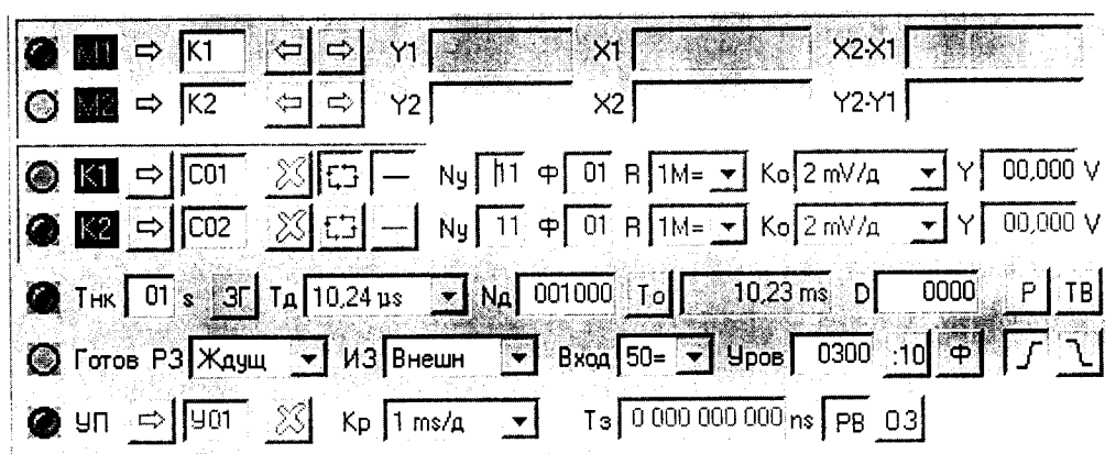
Рисунок 6 – Начальные положения органов управления на панели управления «УИ К2-76 ЦО НЧ» поверяемой установки при определении абсолютной погрешности измерений напряжения каждого из каналов ЦО НЧ поверяемой установки
