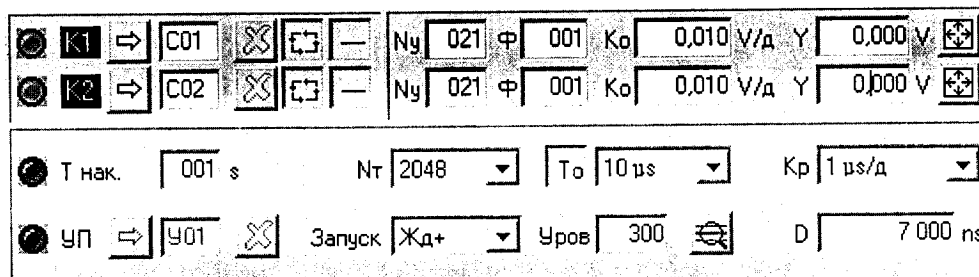
Рисунок 2 – Начальные положения органов управления на панели управления «УИ К2-76 ЦО ВЧ» при измерении абсолютной погрешности измерений напряжения в режиме «ЦО ВЧ» поверяемой установки
