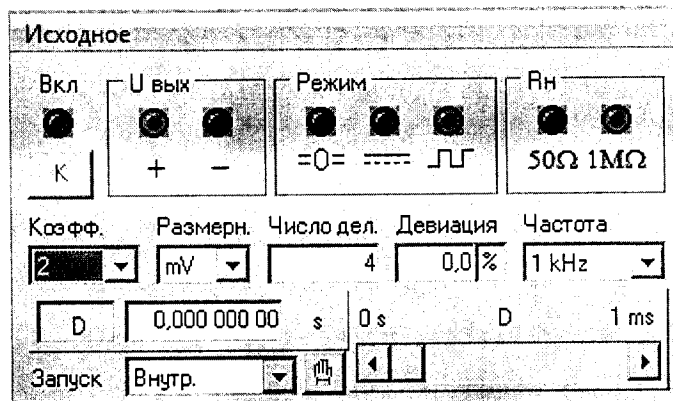
Рисунок 5 – Начальные положения органов управления на панели управления «УИ К2С-62А КУ» при определении абсолютной погрешности измерений напряжения каждого из каналов ЦО НЧ поверяемой установки
