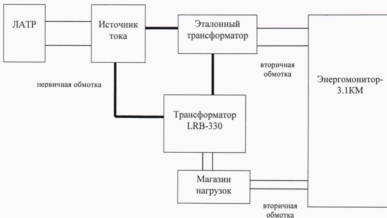
Рисунок 2 – Схема определения метрологических характеристик вторичных обмоток класса точности 0,2S
