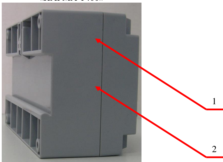
Рисунок 2 – Тыльная панель преобразователя измерительного многофункционального «ПАРМА Т400»
