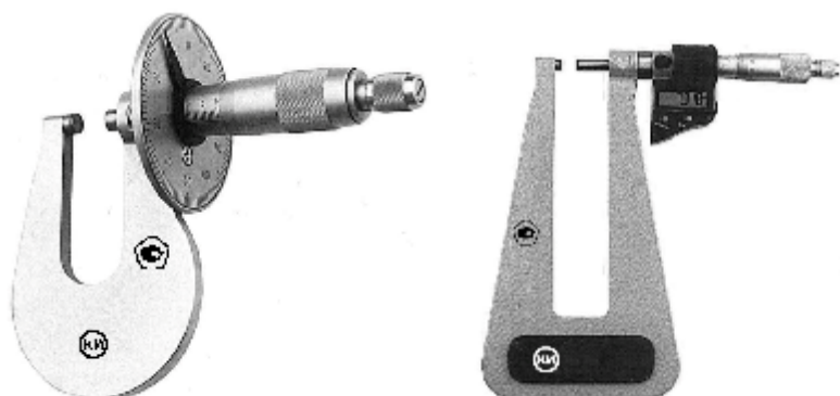
Рисунок 3 – Общий вид микрометров МЛ, МЛ Ц
