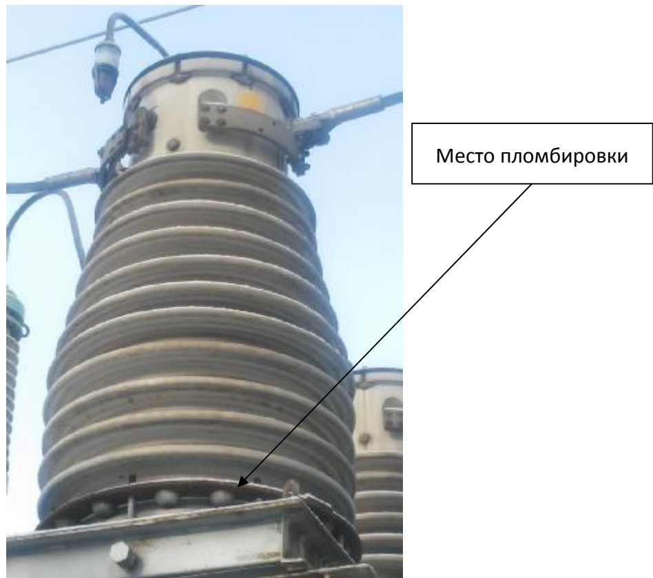
Рисунок 1 – Общий вид трансформатора тока и схема пломбировки от несанкционированного доступа
