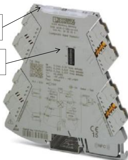
Рисунок 2 - Общий вид преобразователей модификаций MINI MCR-2-UNI-UI-2UI, MINI MCR-2-UNI-UI-2UI-PT, MINI MCR-2-UNI-UI-2UI-C, MINI MCR-2-UNI-UI-2UI-PT-C с указанием мест нанесения знака поверки и пломбирования
