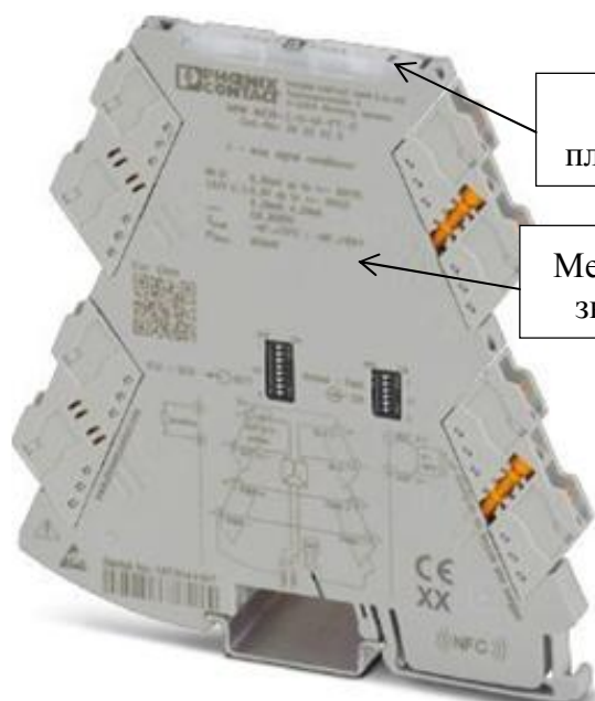
Рисунок 1 - Общий вид преобразователей модификаций MINI MCR-2-U-UI, MINI MCR-2-U-UI-PT, MINI MCR-2-U-UI-C, MINI MCR-2-U-UI-PT-C с указанием мест нанесения знака поверки и пломбирования
