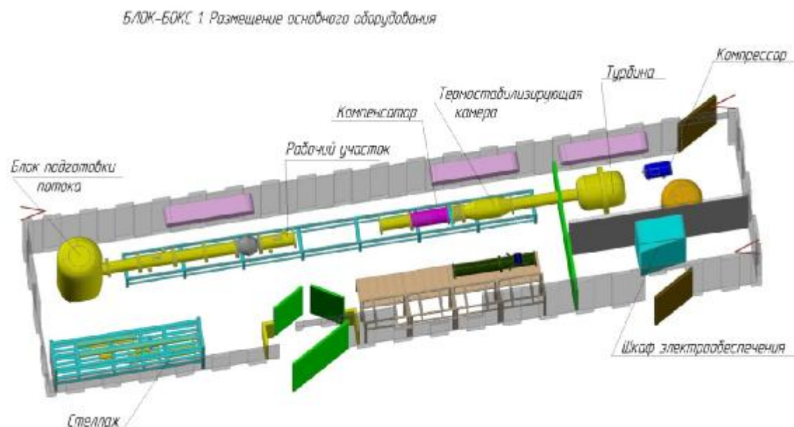
Рисунок 3 – Установка АПУ-Г-110/650М
