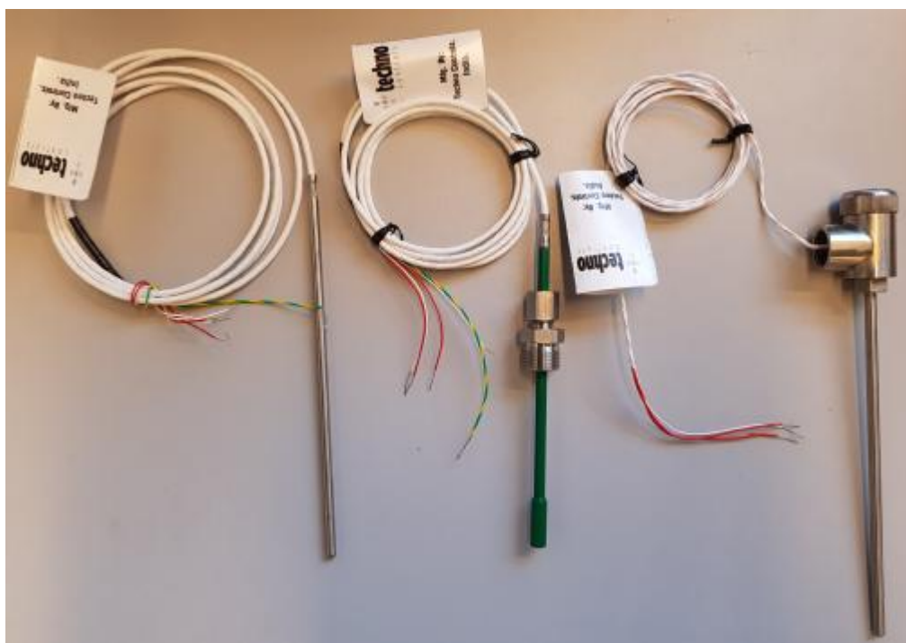
Рисунок 1 – Общий вид ТС (слева направо: ТВТД-О, ТВТД-Л, ТВТД-К)
