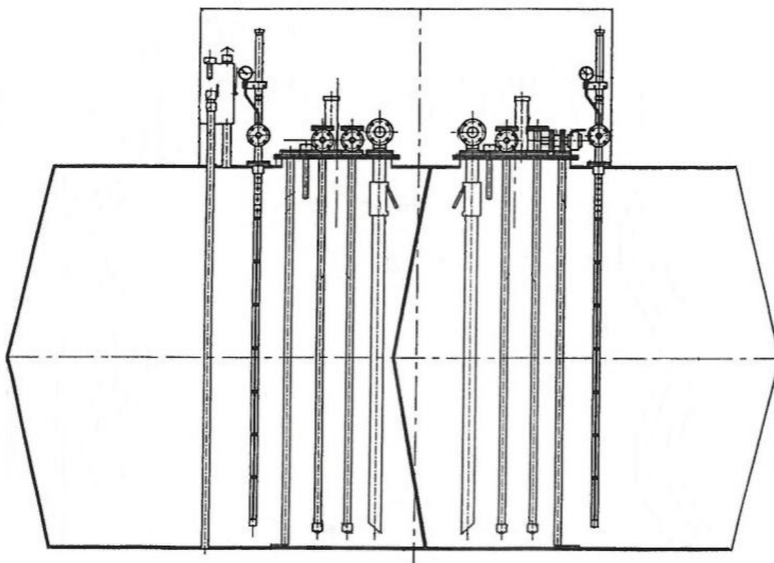
Рисунок 1 – Эскиз резервуаров РГС-25
