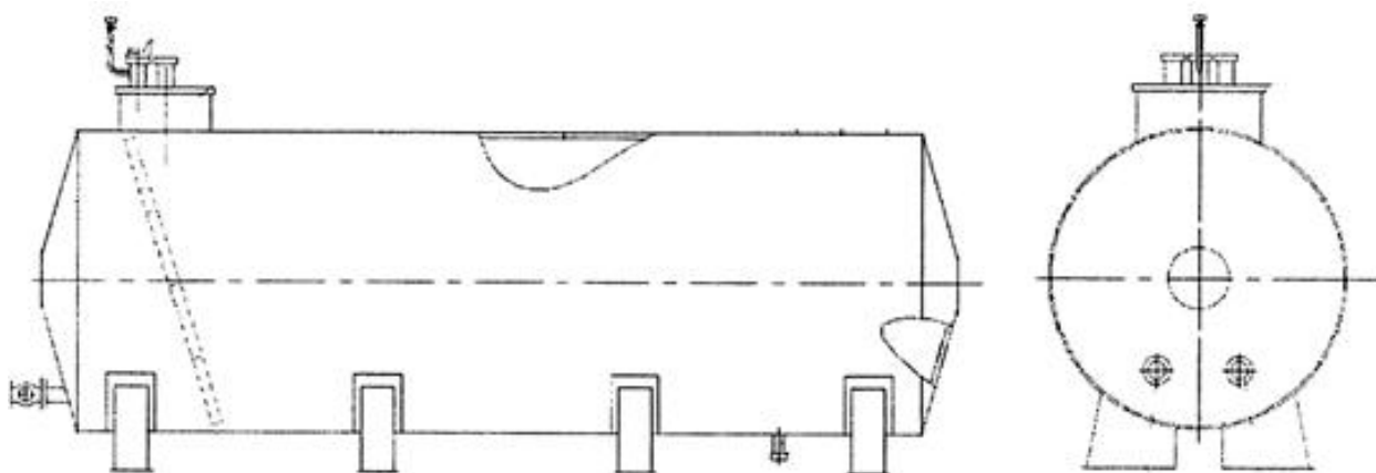
Рисунок 1 – Эскиз резервуара стального горизонтального цилиндрического РГС-50
