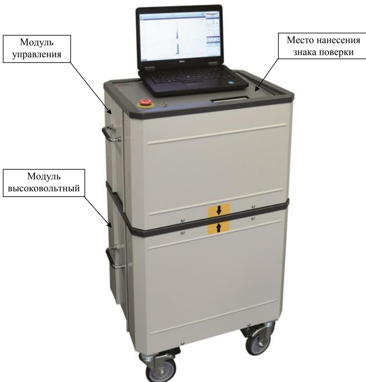
Рисунок 1 – Общий вид систем MV DAC-30
