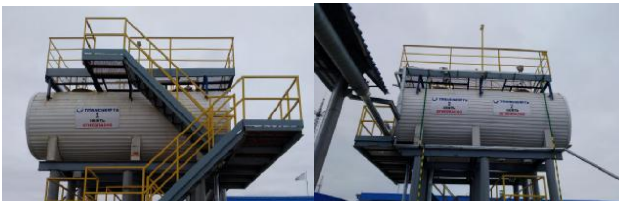
Рисунок 1 – Общий вид РГС
