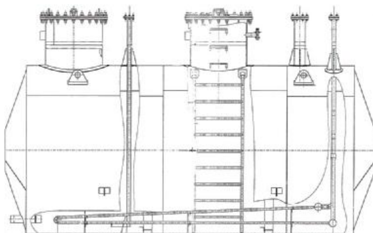
Рисунок 2 – Эскиз резервуара РГС-20
