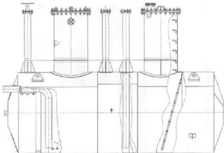
Рисунок 1 – Эскиз резервуара РГС-16
