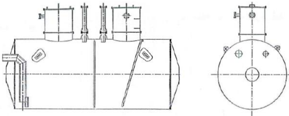
Рисунок 1 – Эскиз резервуара РГС-20
