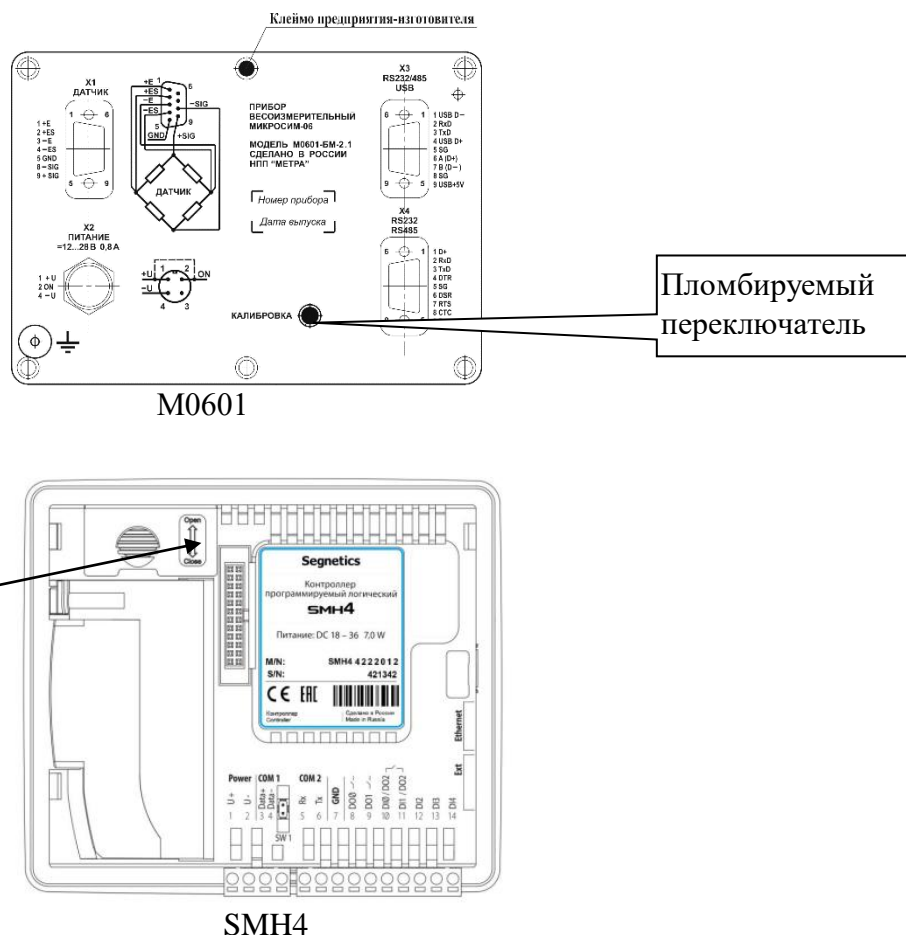
Рисунок 3 – Схема пломбировки от несанкционированного доступа и обозначение мест нанесения знака поверки
