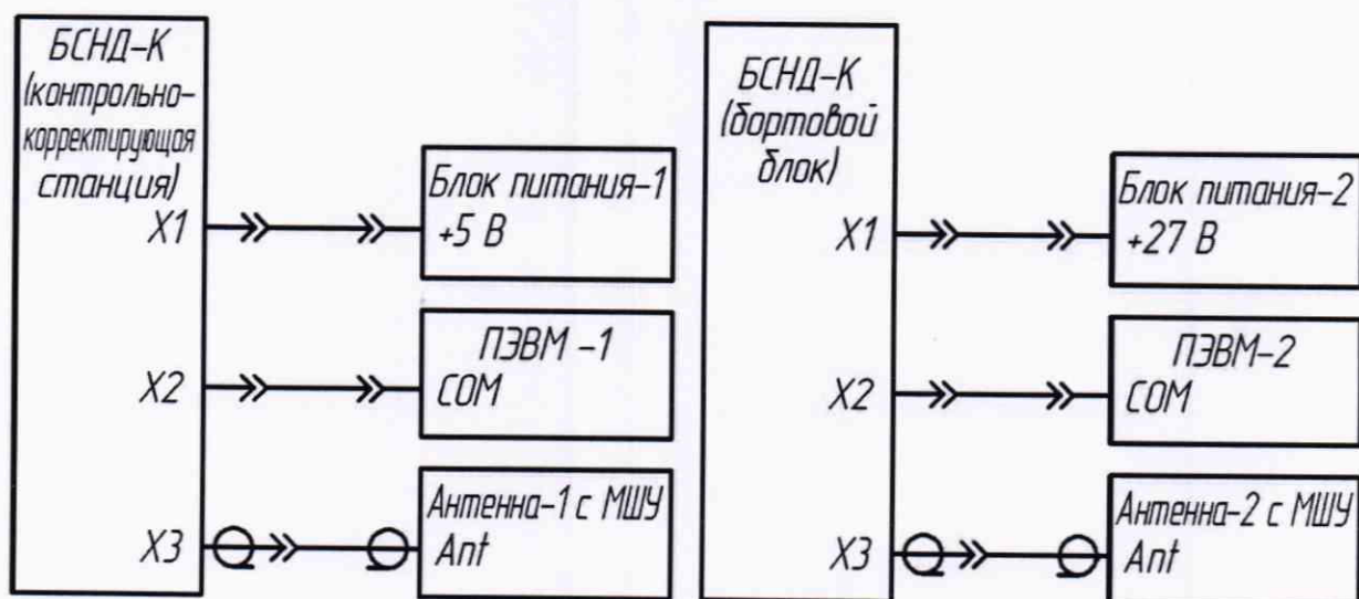
Рисунок 3 — Схема подключения бортового устройства ГН при определении координат
