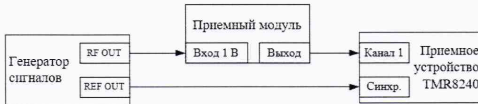
Рисунок 1 – Схема подключения
