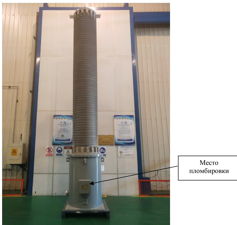
Рисунок 4 – Общий вид трансформаторов исполнения JDQXF-500 с указанием места пломбирования от несанкционированного доступа
