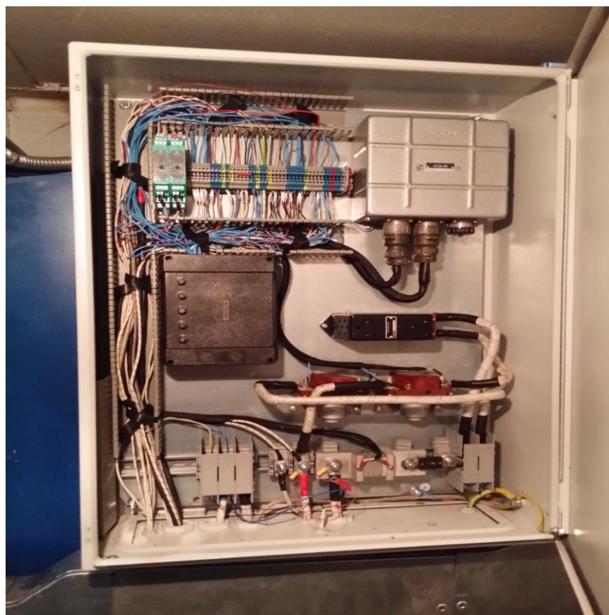
Рисунок 6 - Шкаф запуска
