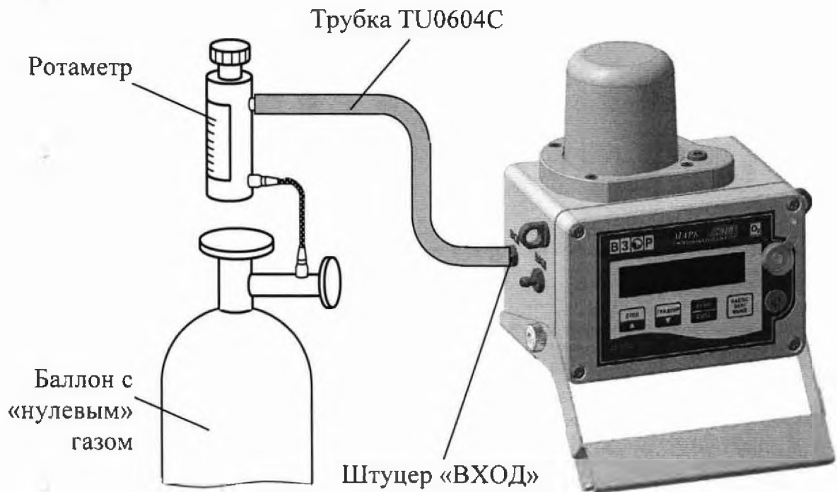
Рисунок 2.3 – Проверка реакции датчика на кислород с помощью «нулевого» газа
