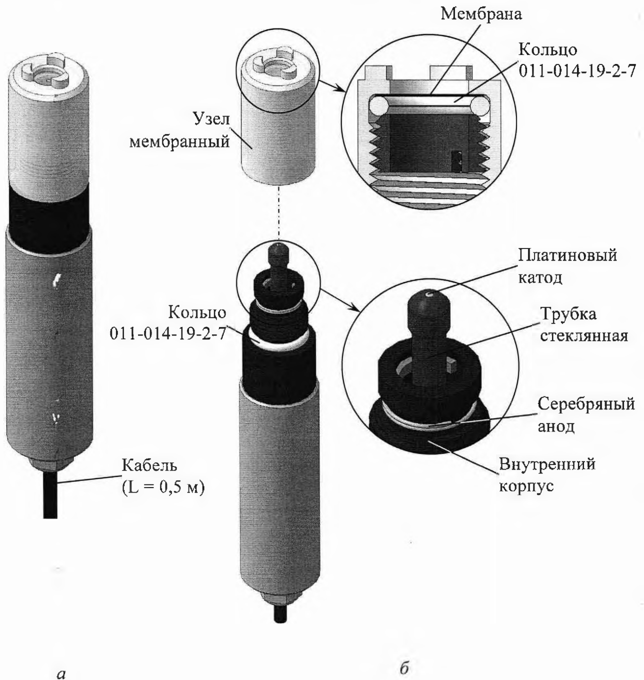
Рисунок 1.3 – Датчик кислородный ДК-2010
