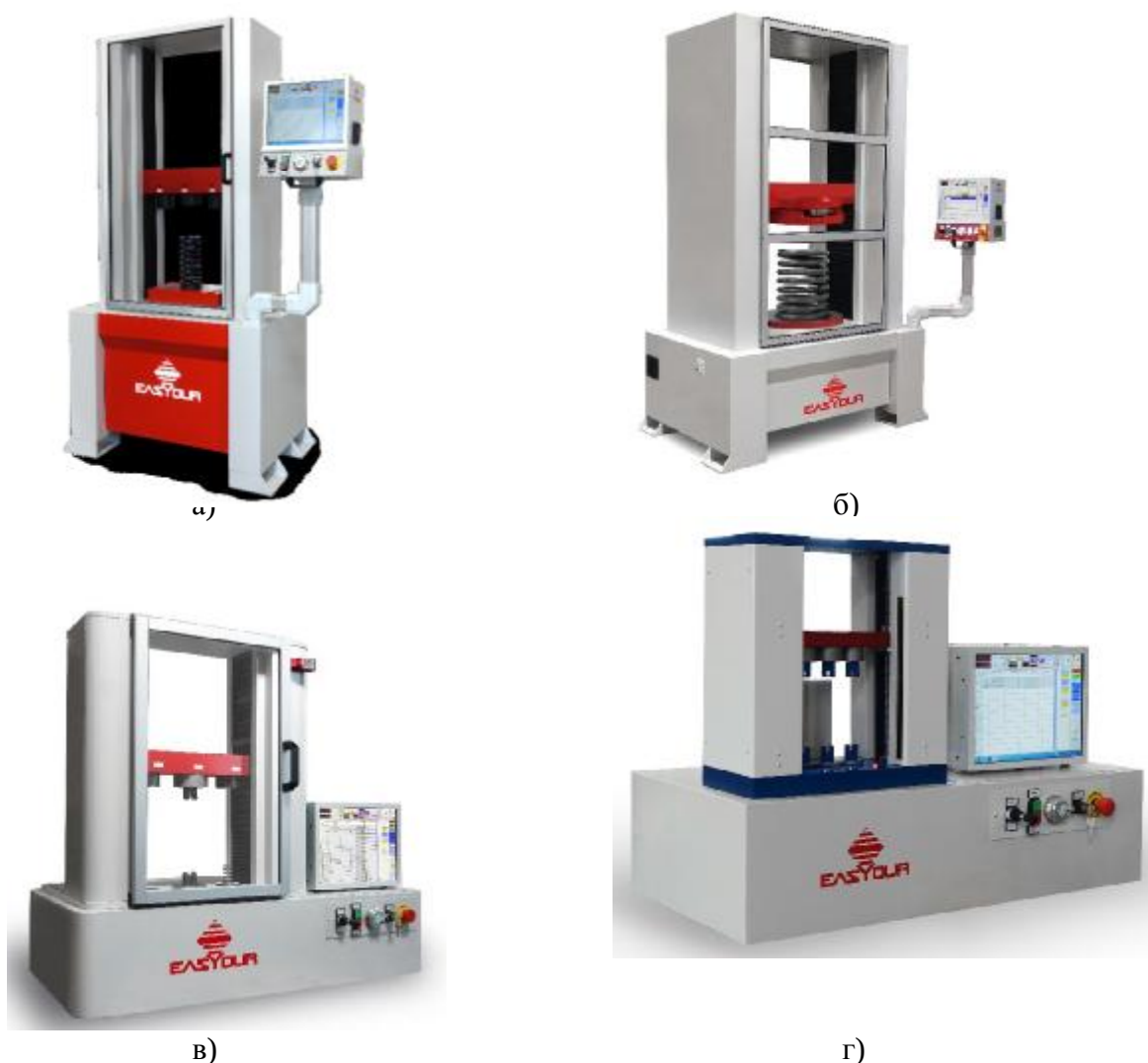
Рисунок 1 – Общий вид машин испытательных EASYDUR а) 3MZ1 TRIPLE, 3MZ2.5 TRIPLE, 3MZ5 TRIPLE; б) AURA10, AURA30, AURA60, AURA100; в) DYNO TRIPLE; г) MICRODYNO TRIPLE
