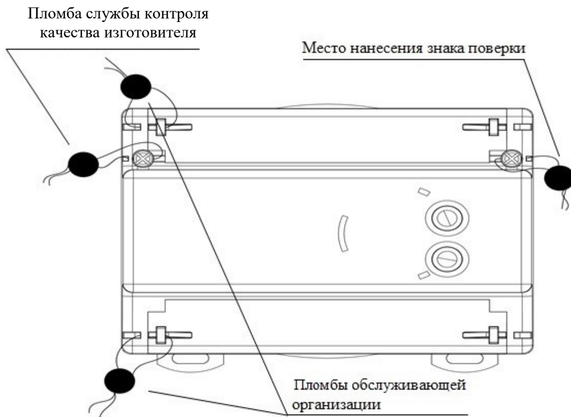
Рисунок 1 - Общий вид счётчиков
