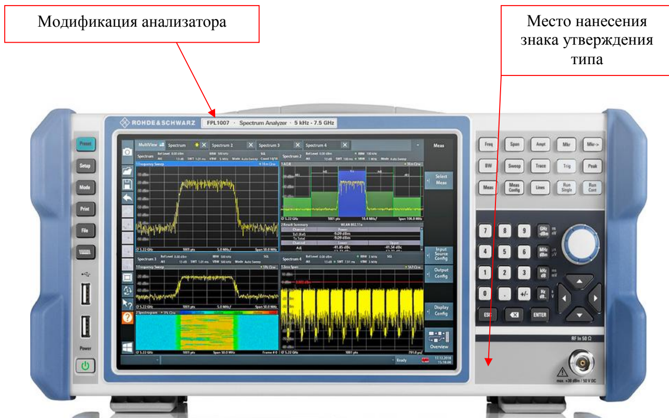
Рисунок 1 - Общий вид анализаторов спектра FPL1003, FPL1007
