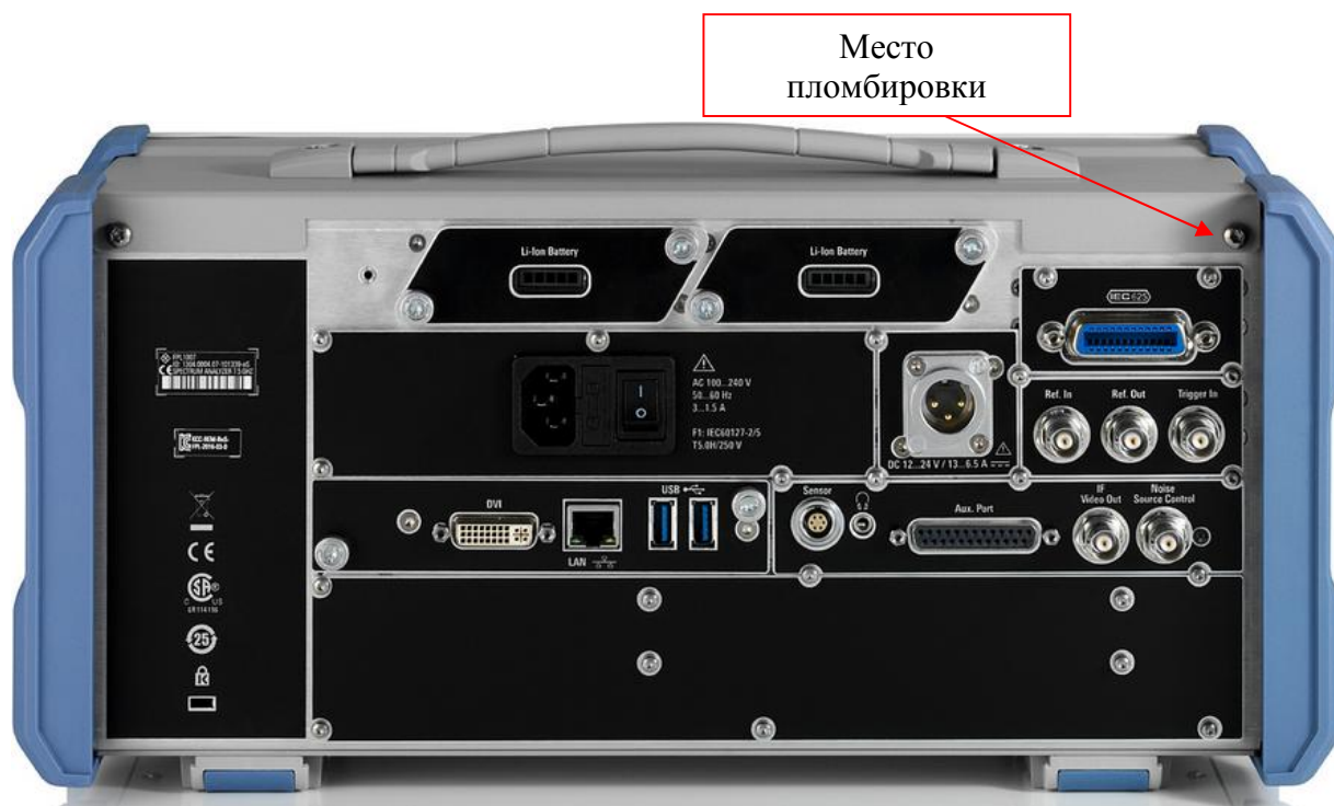
Рисунок 2 - Схема пломбировки анализаторов спектра FPL1003, FPL1007 от несанкционированного доступа
