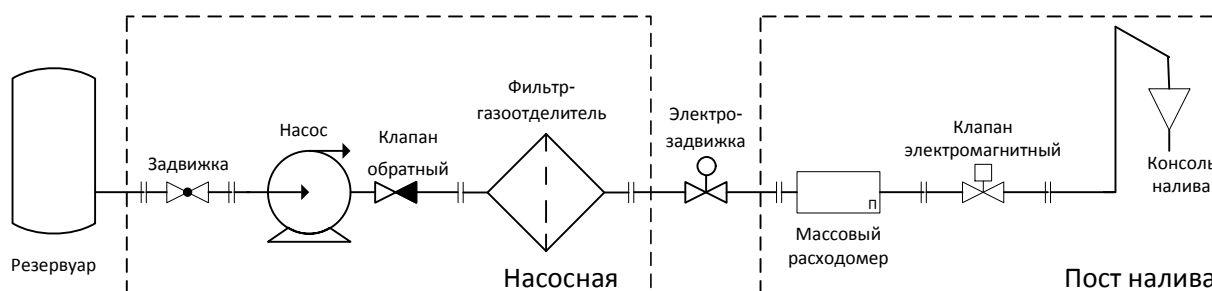
Рисунок 2 – Принципиальная схема поста налива
