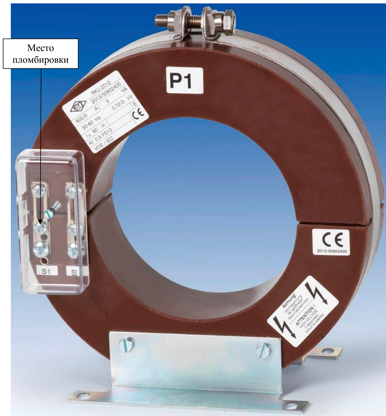
Рисунок 2 – Общий вид трансформаторов тока RKU
