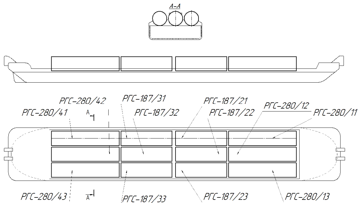
Рисунок 1 - Общий вид, номера и расположение резервуаров на барже проекта КН16801
