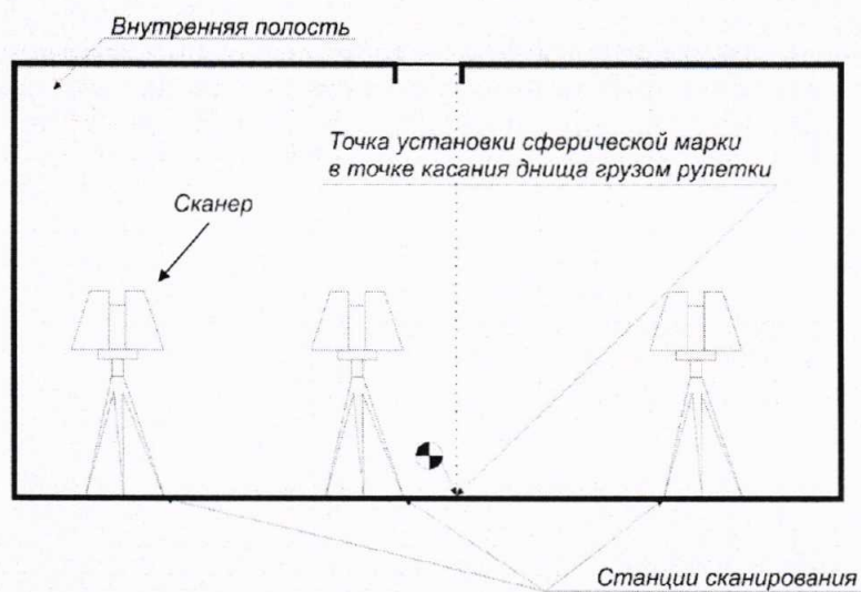
Рисунок А.2 – Схема сканирования внутренней полости резервуара
