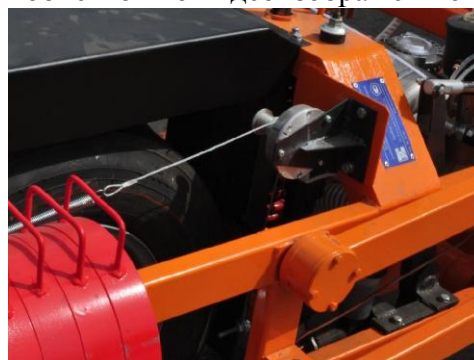
Рисунок 18 – Толкочмер РДТ-811 канала измерений амплитуды колебаний подвески прибора ПКРС
