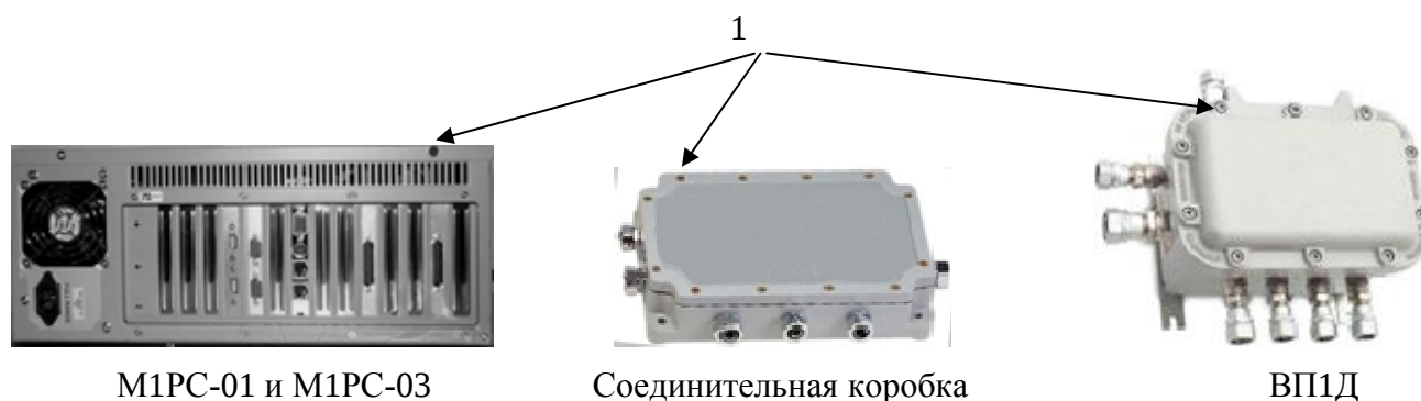
Рисунок 3 – Схема пломбировки от несанкционированного доступа (где 1 – мастичная пломба)
