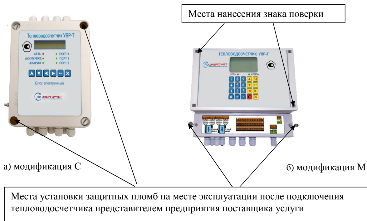
Рисунок 6–Места пломбирования тепловосчетчиков УВР-Т
