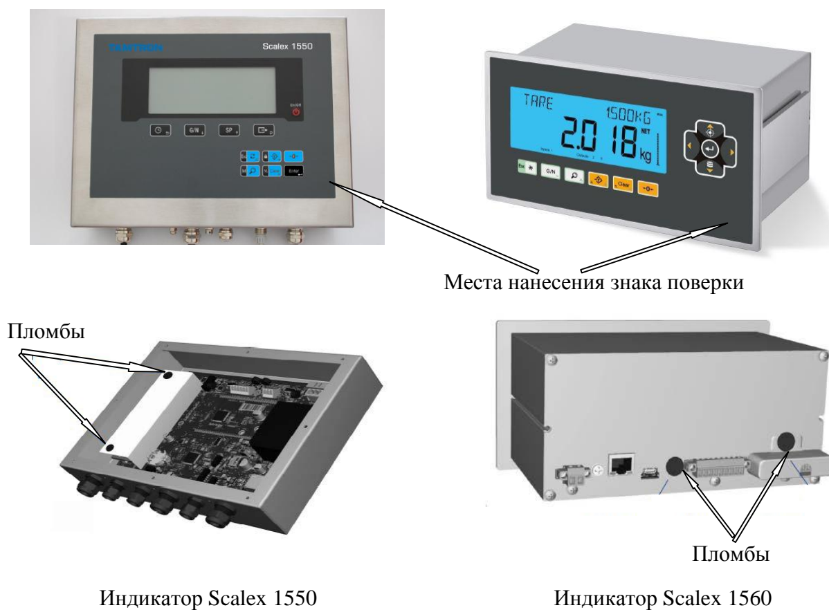
Рисунок 3 – Общий вид индикаторов, схем пломбировки индикаторов и обозначение мест нанесения знака поверки
