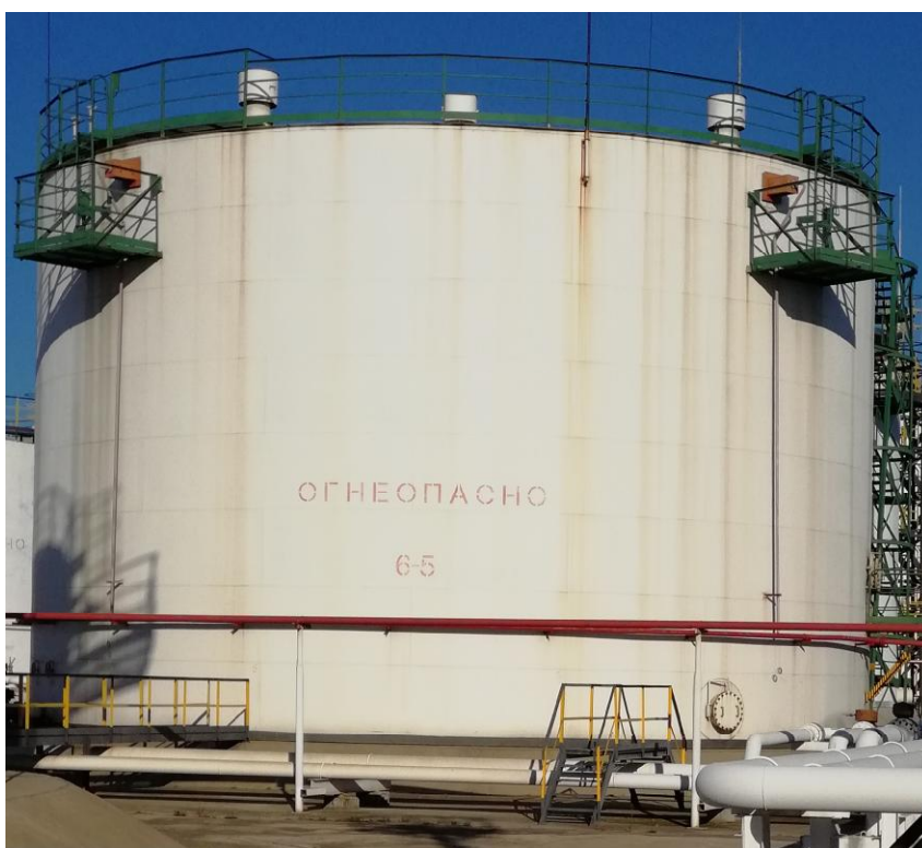
Рисунок 5 - Общий вид резервуара стального вертикального цилиндрического RVSP-3000
