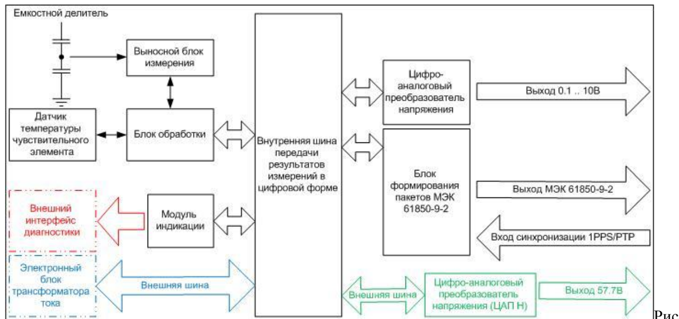
Рисунок 1 – Блок-схема ДНЕЭ
