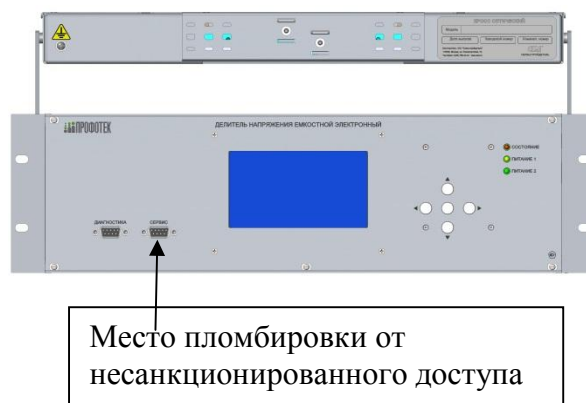
Рисунок 3 – Общий вид электронного блока ДНЕЭ (вид спереди) и схема пломбировки от несанкционированного доступа
