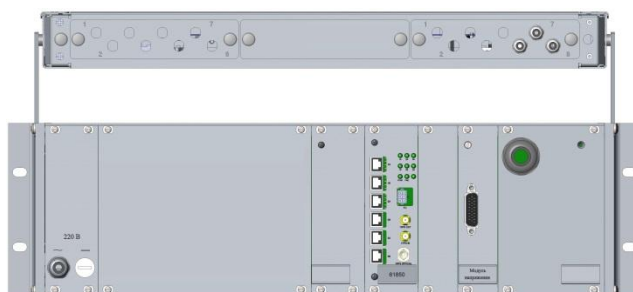
Рисунок 4 – Общий вид электронного блока ДНЕЭ (вид сзади)
