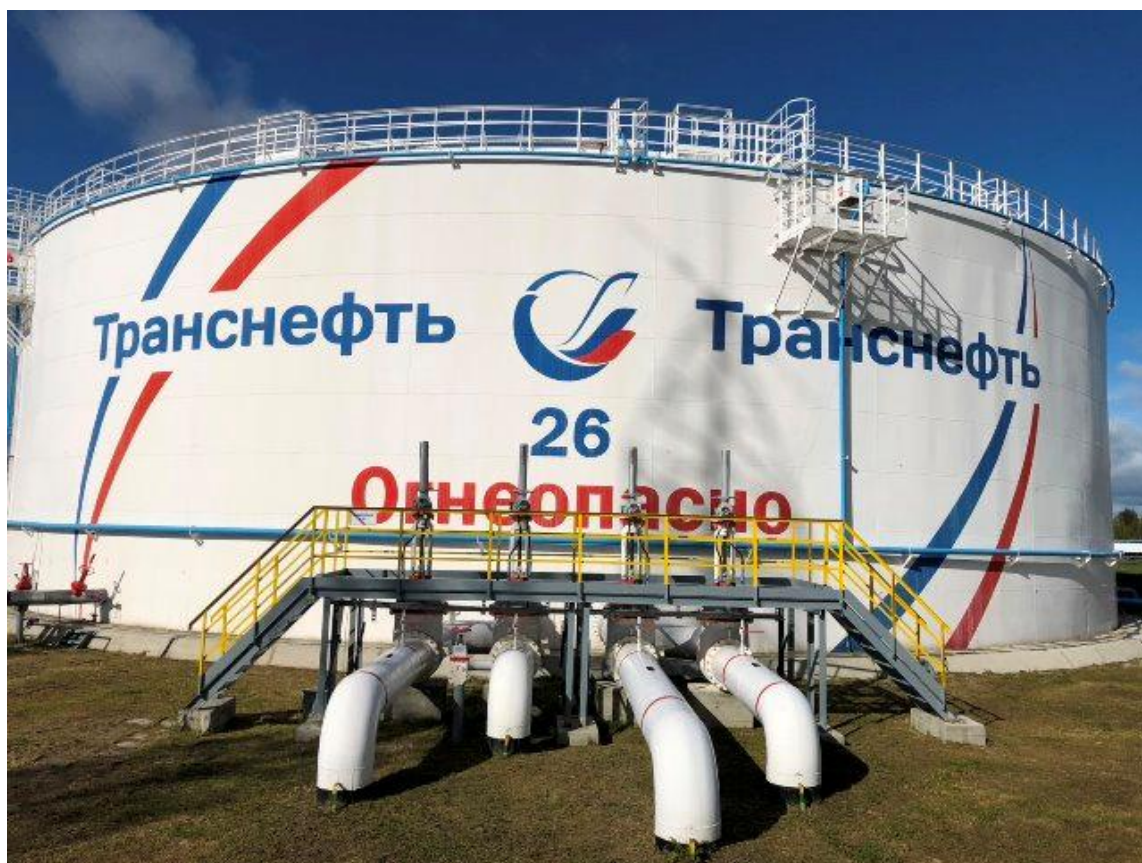
Рисунок 3 - Общий вид резервуара вертикального стального цилиндрического РВСП-20000
