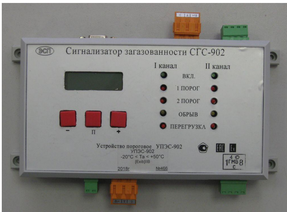
а) устройство пороговое двухканальное УПЭС-902
