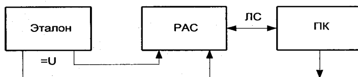
Рисунок 1 — Схема соединений для определения приведенной к верхнему пределу измерения погрешности измерения постоянного напряжения
