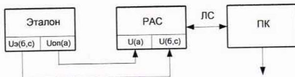
Рисунок 7 - Схема соединений для определения абсолютной погрешности измерения угла фазового сдвига между напряжениями разных фаз
